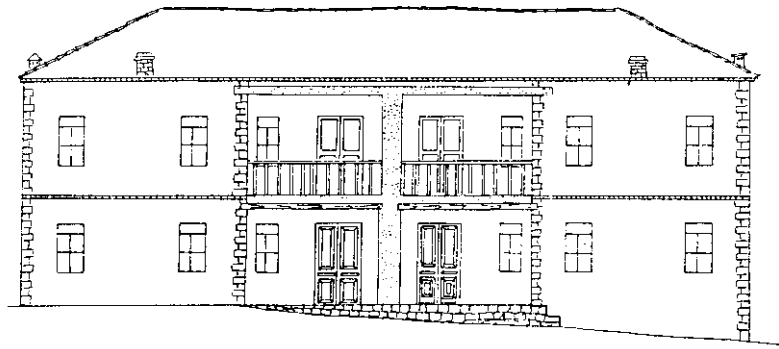
Figure 6. Planimétrie d'un autre type de maison dans le village de Lumalas
