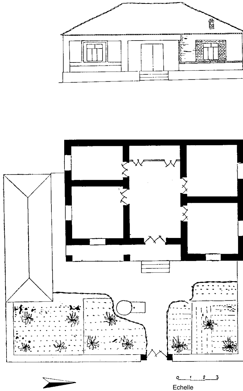
Figure 5. Planimétrie d'une maison dans le village de Lumalas
